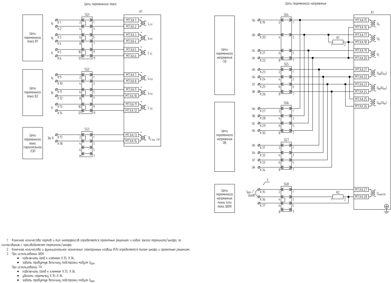
Рисунок Г.1 – Схема электрическая принципиальная (часть 1)
