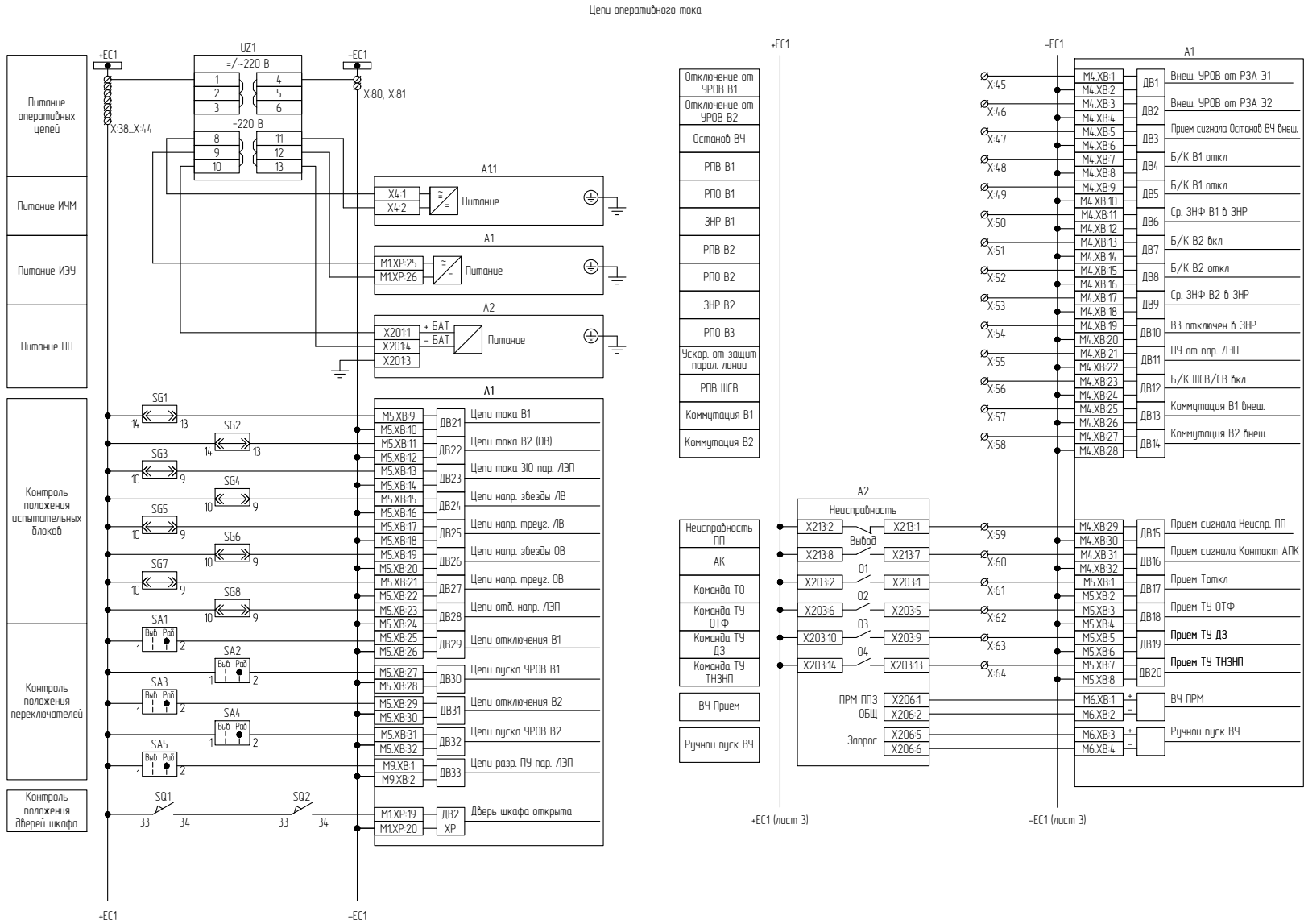
Рисунок Г.2 – Схема электрическая принципиальная (часть 2)
